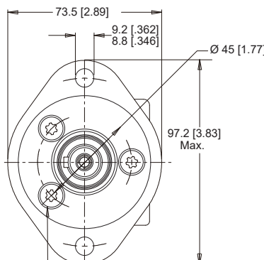
LKB - (3) M6 x 1, Min. Depth 10 [.394] LL5 - (3) 1/4-28 UNF, Min. Depth 10 [.394]
